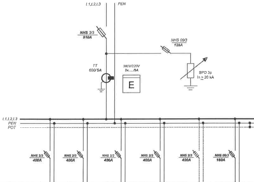
Табло за МПТ до 400 kVA
