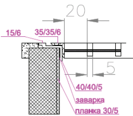
Детайл "А"
