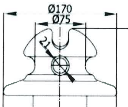
3. Чертеж на горната част на изолатор ИНК или NS /Zeichnung des oberen Teils von Isolator INK oder NS
