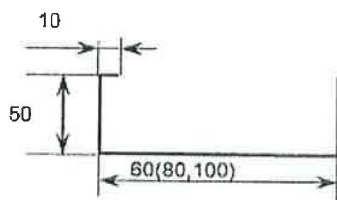
Чертеж 1. - Кабелен канал
