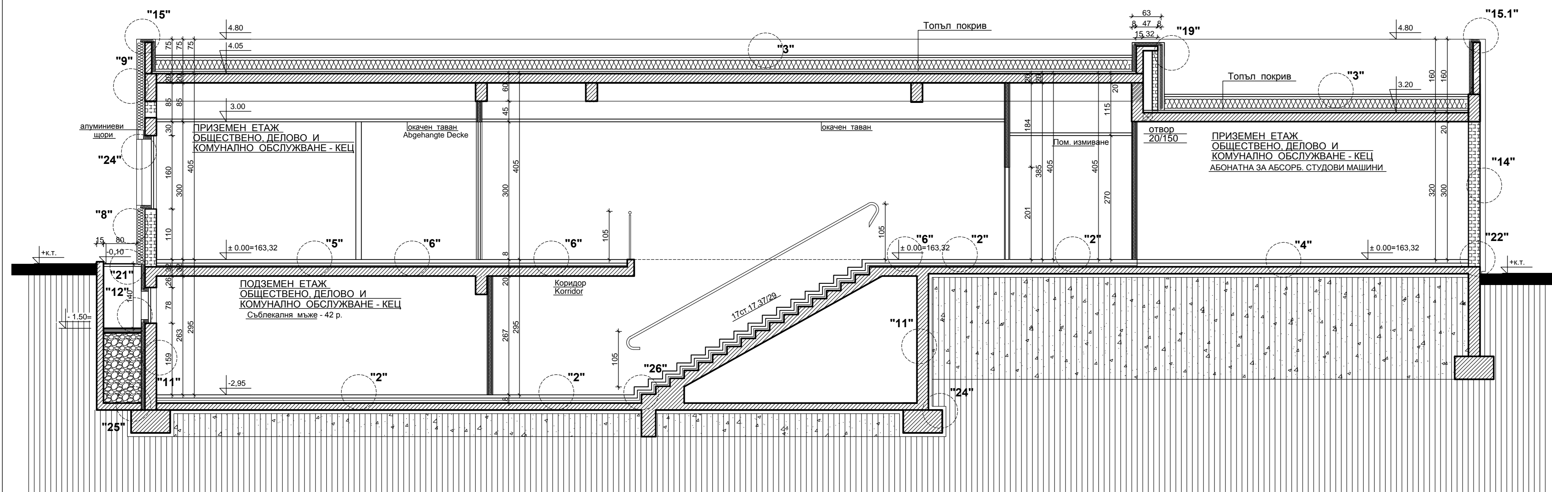
ВЕРТИКАЛЕН РАЗРЕЗ "1-1" М 1: 50
