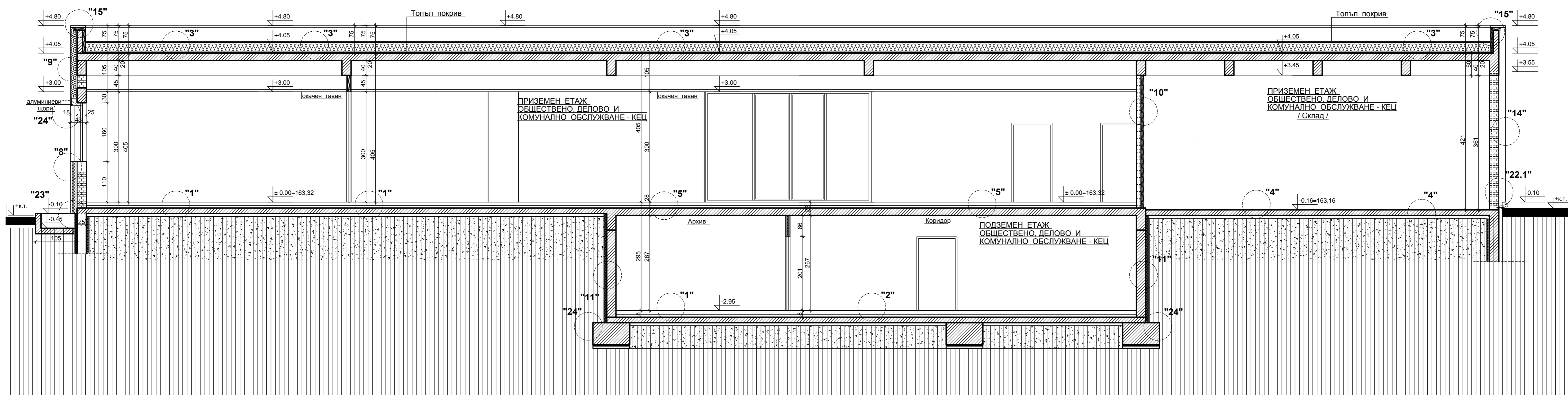
ВЕРТИКАЛЕН РАЗРЕЗ "3-3" М 1: 50
