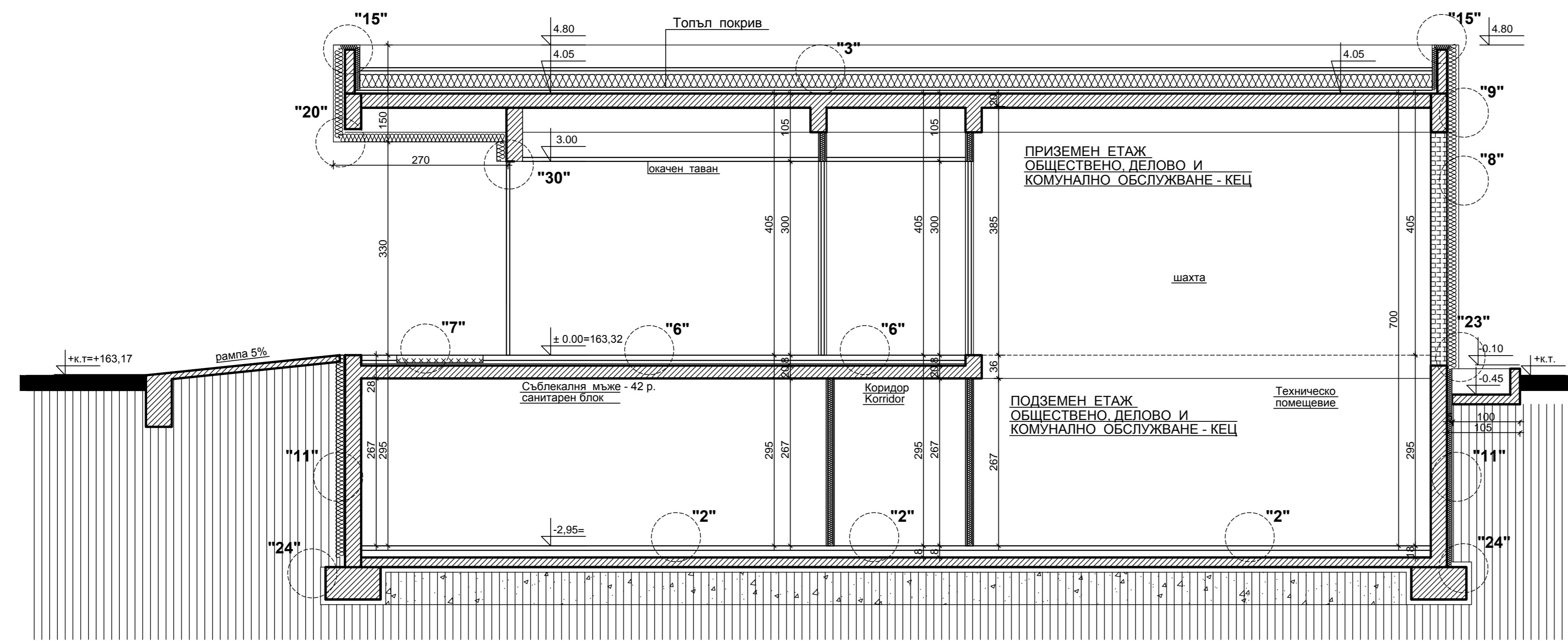
ВЕРТИКАЛЕН РАЗРЕЗ "2-2" М 1: 50
