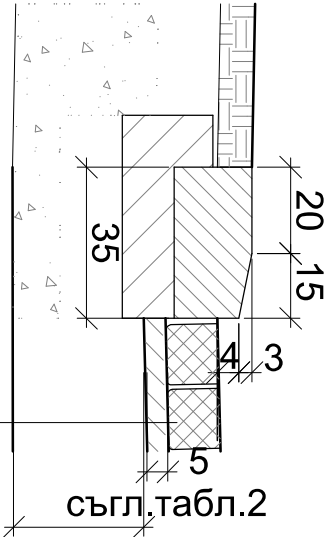
Паваж със заклинен трошен камък
