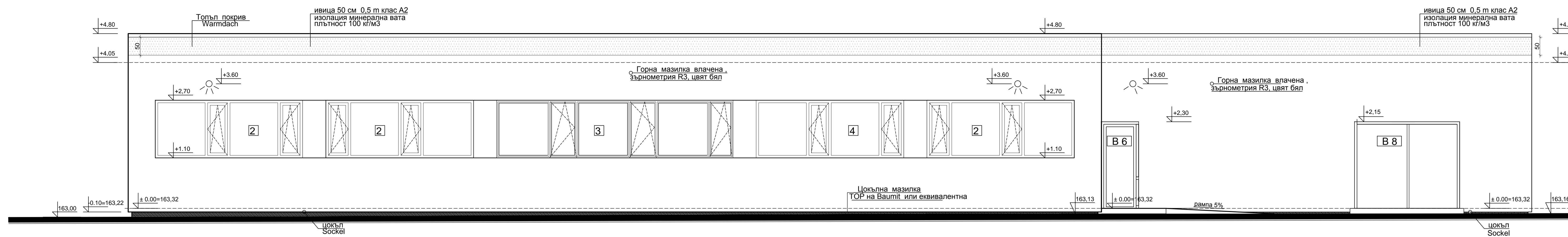
ФАСАДА ЮГОИЗТОК M 1:50
