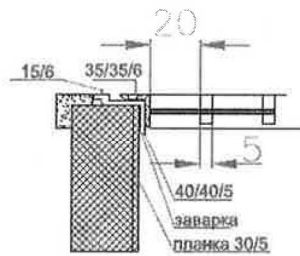
Детайл "А"
