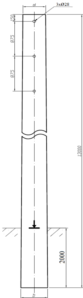
Фигура 1. Двуконпонентен композитен модулен стълб за въздушни електропроводи СрН
