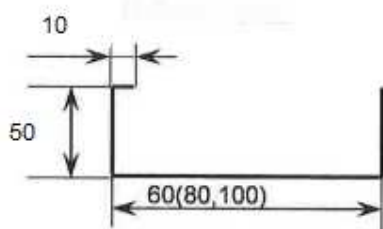
Чертеж 1. - Кабелен канал
