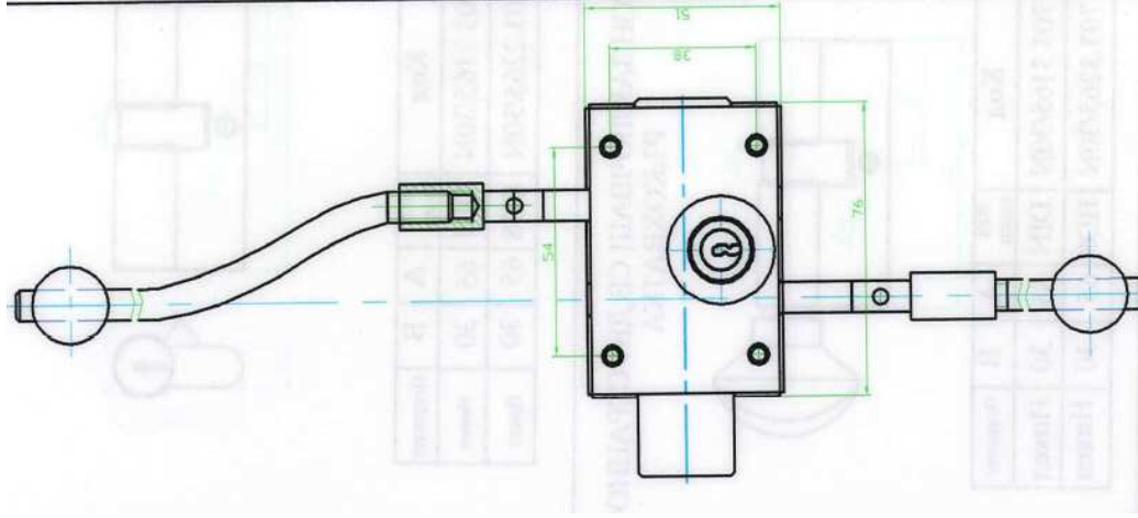
Чертеж на секретна брава / Zeichnung des Sicherheitsschlusses
