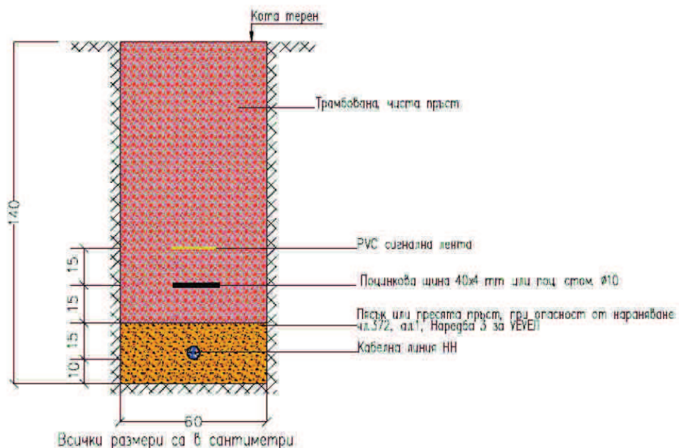
Пологане на кабел НН в изкоп в земеделска земя с пясъчна възглавница
