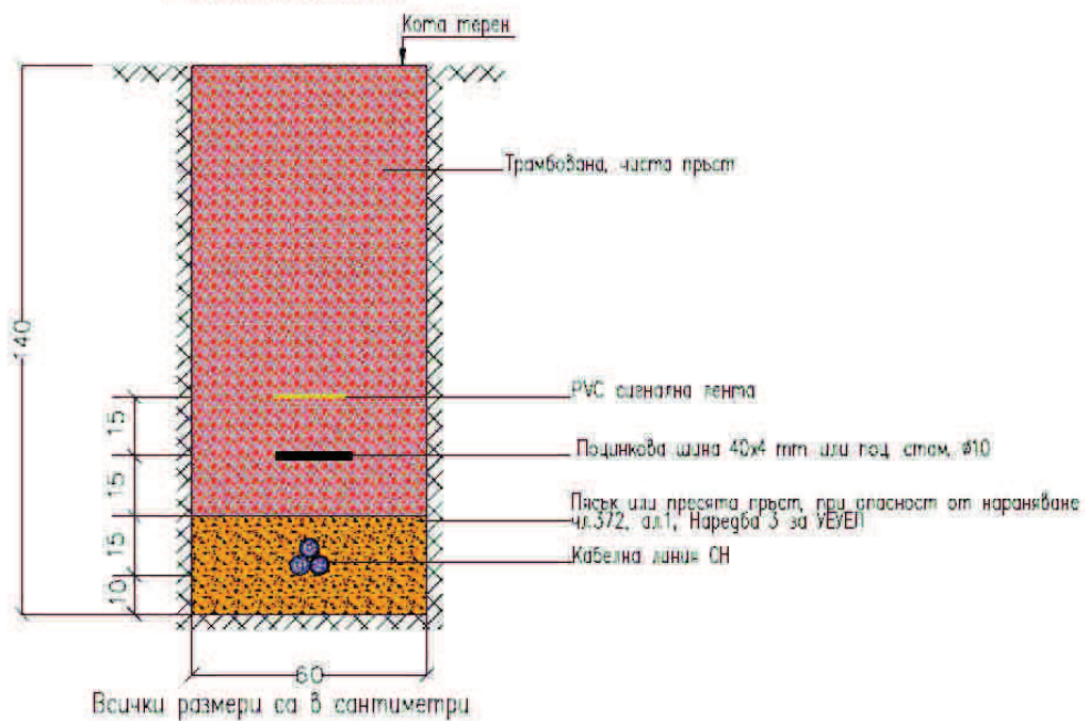
Пологане на кабел СрН в изкоп в земеделска земя с пясъчна възглавница
