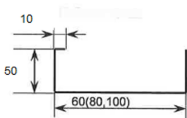
Чертеж 1. - Кабелен канал
