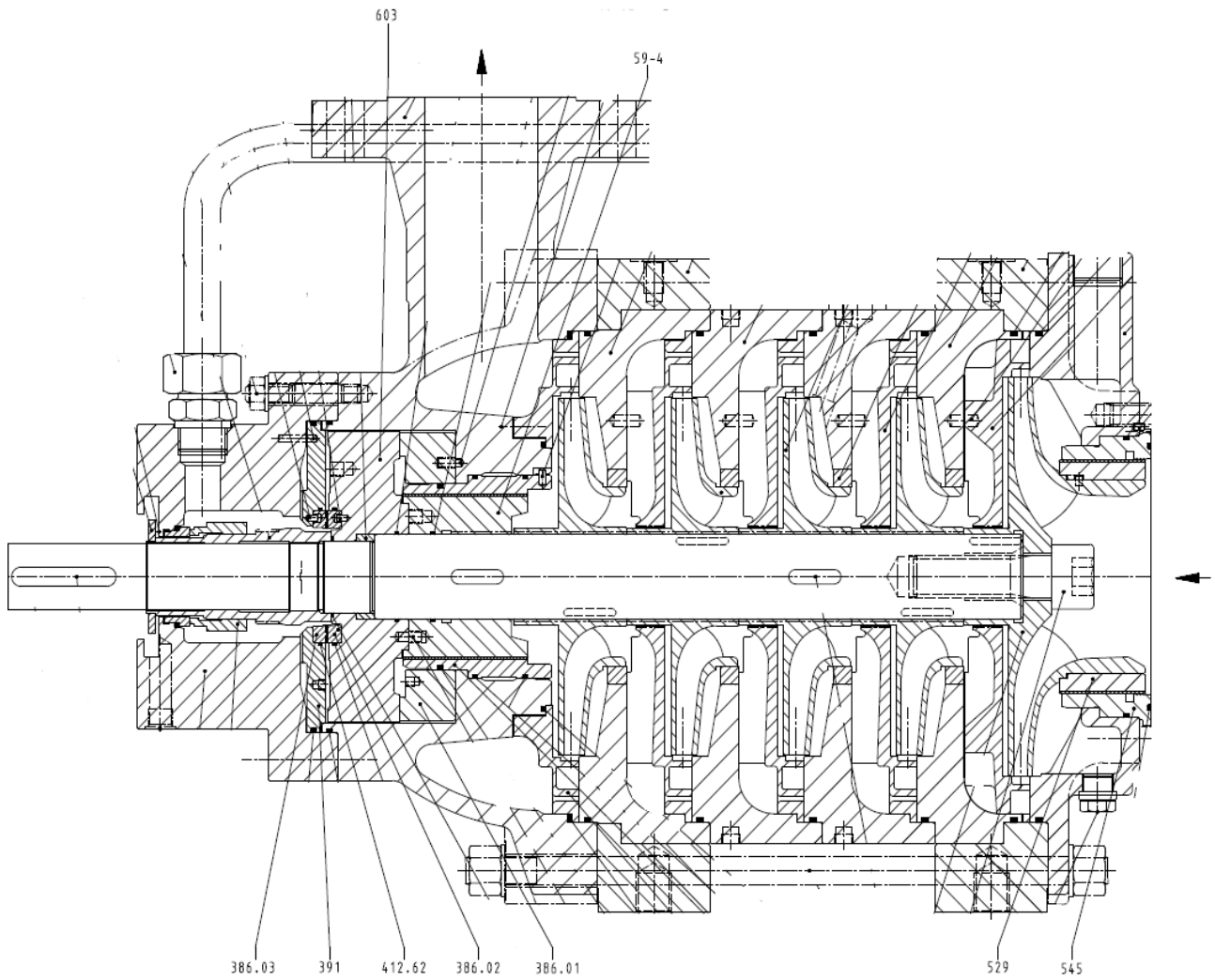
Схема детали помпа тип HGM 2/11
