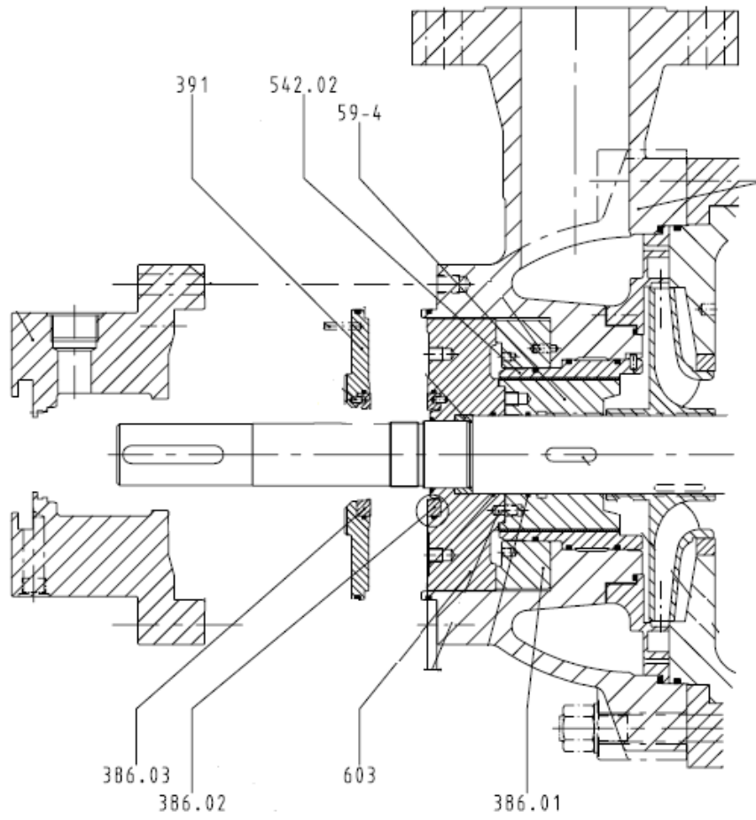
Лагерен възел помпа, край към електро двигател
