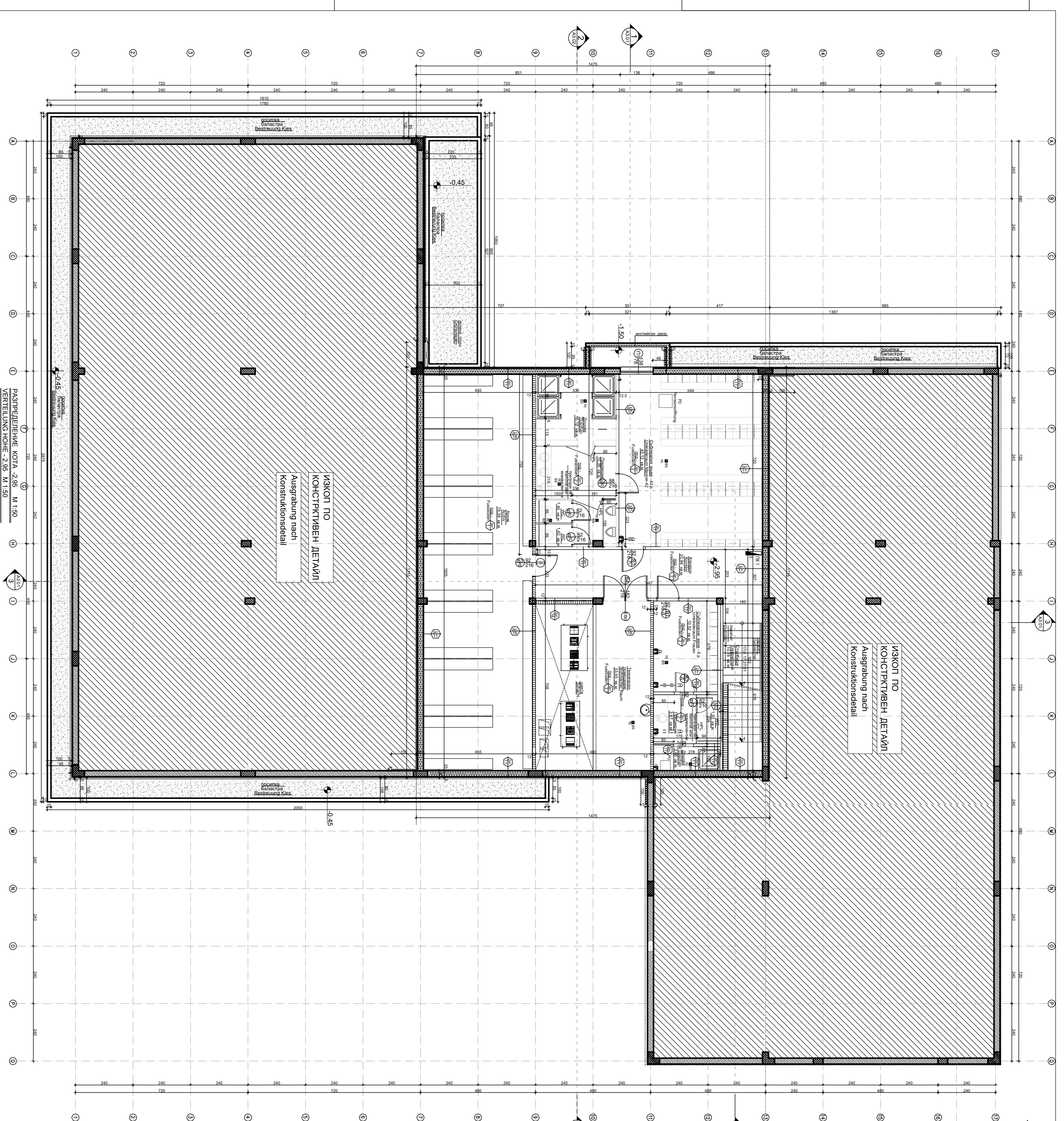
ПАСПЕЛЕНИЕ КОТА -2,95 М 1:50 VERTIEBLUNG HOHE -2,95 М 1:50
